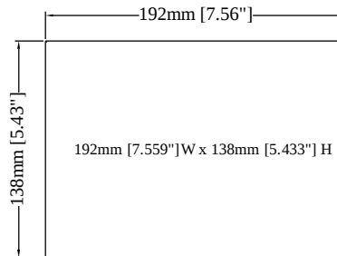
Cutout Dimensions
