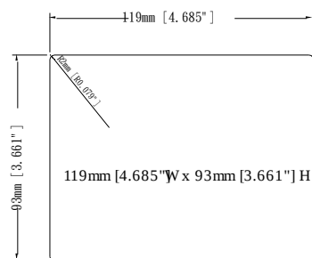
Cutout Dimensions
